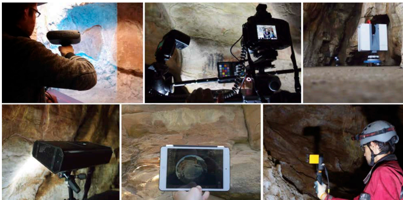
Fig. 3 Diferentes sistemas de documentación tridimensional aplicados en conjuntos rupestres
