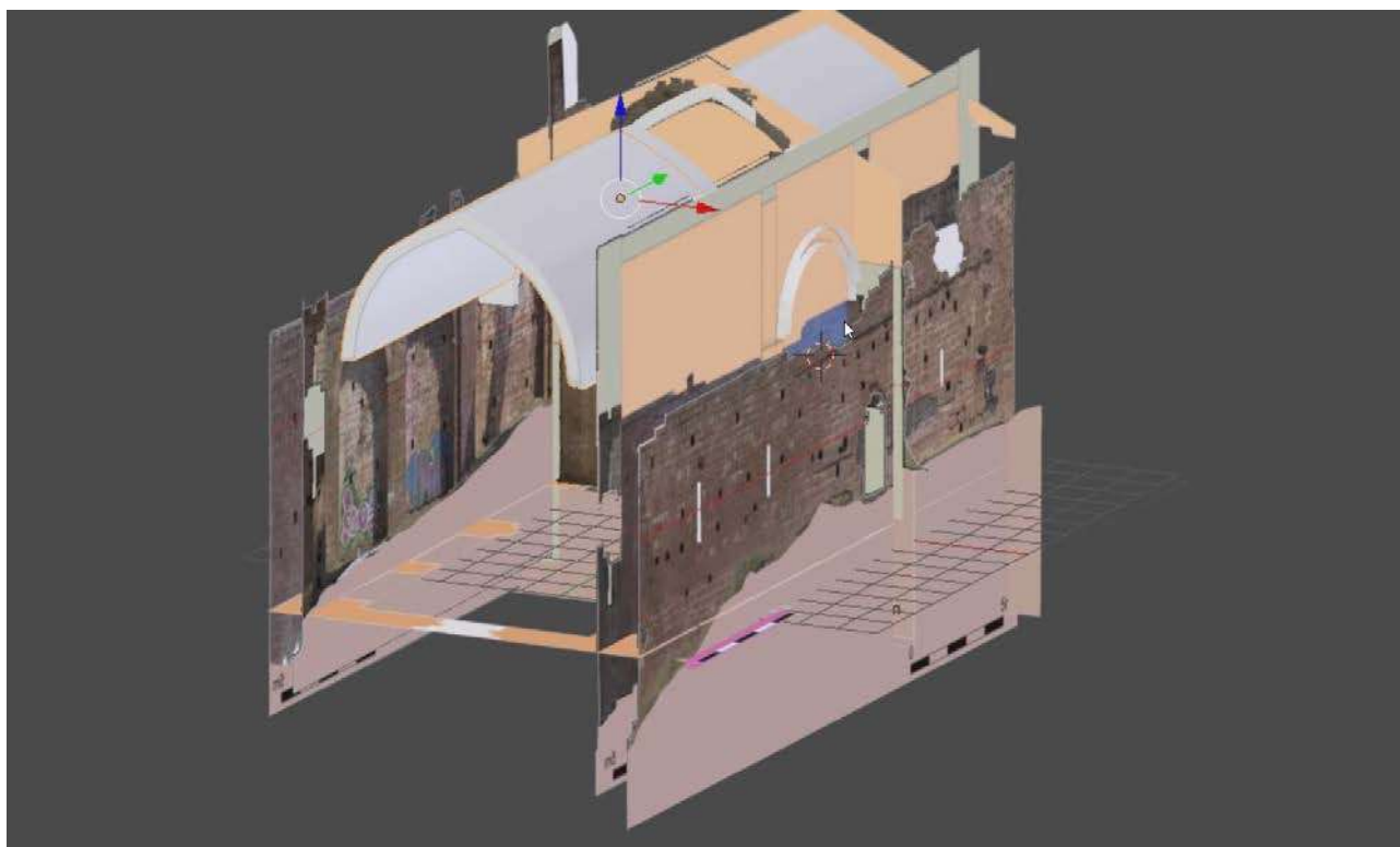
Fig. 3 Proceso de construcción del modelo de la iglesia de Sant Genís de Rocafort a partir de las distintas fuentes de información
