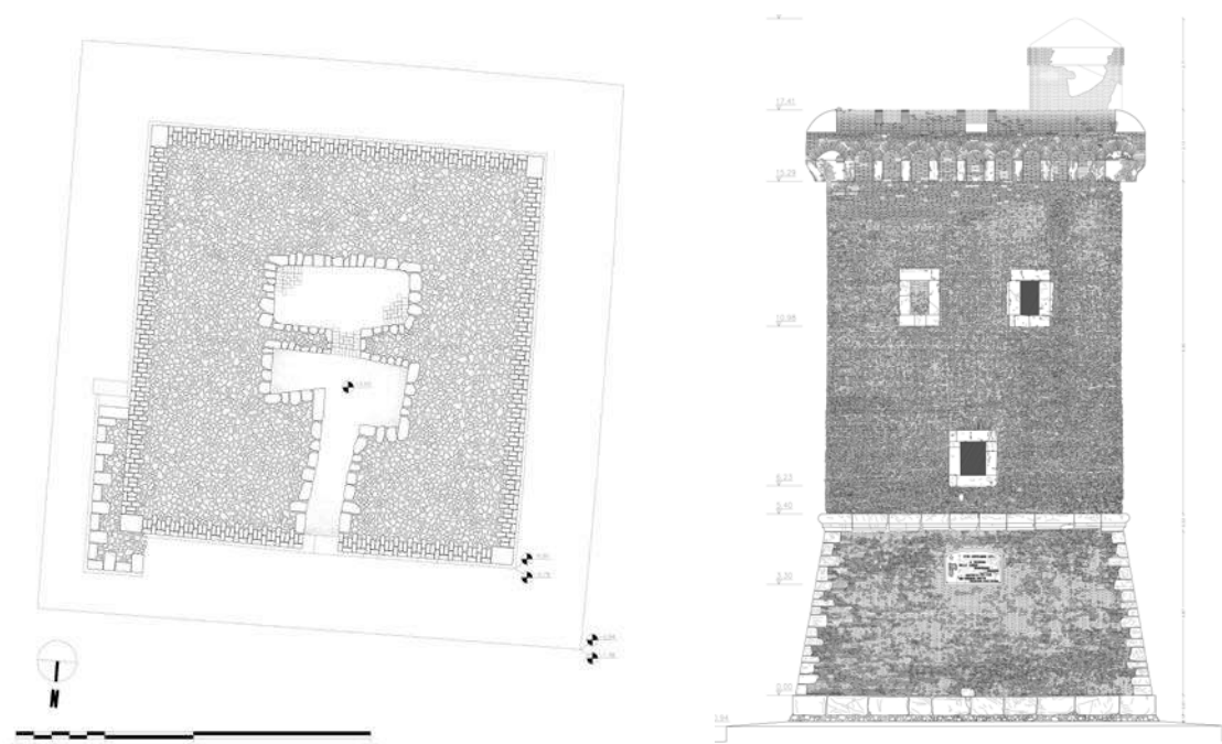
Fig. 3 Torre Olevola (S. Felice Circeo), levantamiento, planta y alzado 1/200
