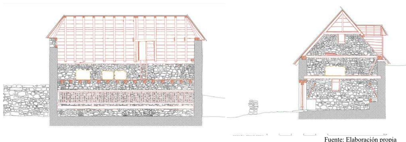
Fig. 4 Sección longitudinal y transversal de la borda de casa La Fon en Las Corcillas
