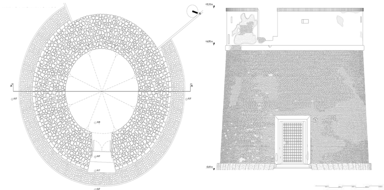
Fig. 4 Torre di Caldano (Anzio), levantamiento, planta y alzado 1/200
