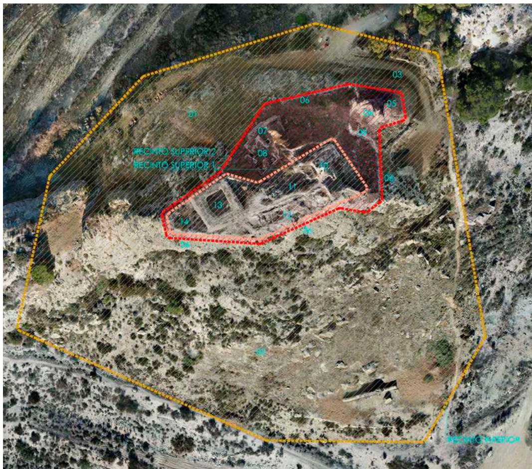
Fig. 7 Elementos del Castell de Tibi: Recinto inferior: 1-Ladera norte, 2-Ladera sur, 3-Foso; Recinto superior 2: 4-Torre Oriental, 5-Plataforma Oriental, 6-Murallas, 7-Aljibe inferior, 8-Estancias septentrionales, 9-Acceso; Recinto superior 1: 10-Aljibe superior, 11-Estancias centrales, 12-Estancias meridionales, 13-Torre principal y 14-Plataforma occidental
