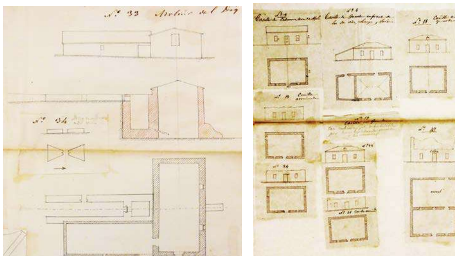
Fig. 2 Detalle del Molino del Dique y planos de las casas de guarda. Año 1880
