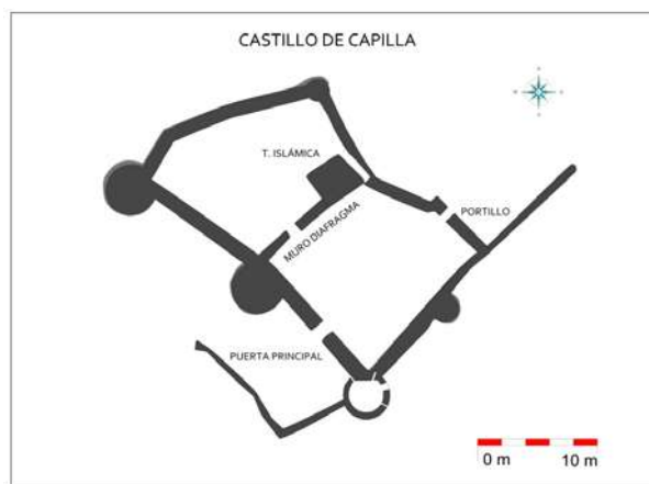
Fig. 1 Planta del castillo de Capilla
