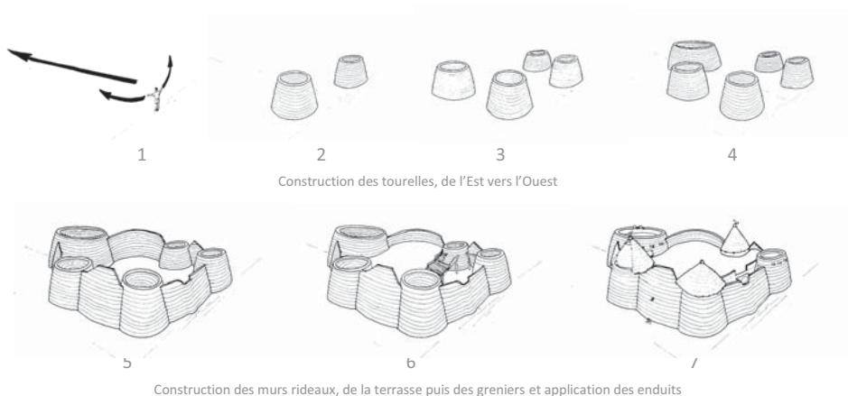
Etapas de construction d'une Takienta (Dessins de Wilfredo Carazas Aedo, CRAterre)
