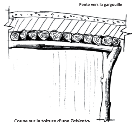
Coupe sur la toiture d'une Takienta .
