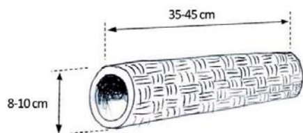
Dimensions courantes d'une gargouille
