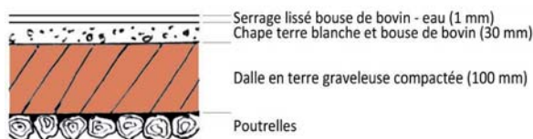
Différentes couches d'une terrasse de takienta
