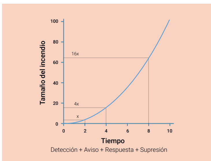
Figura 2. Crecimiento del fuego en función del tiempo
