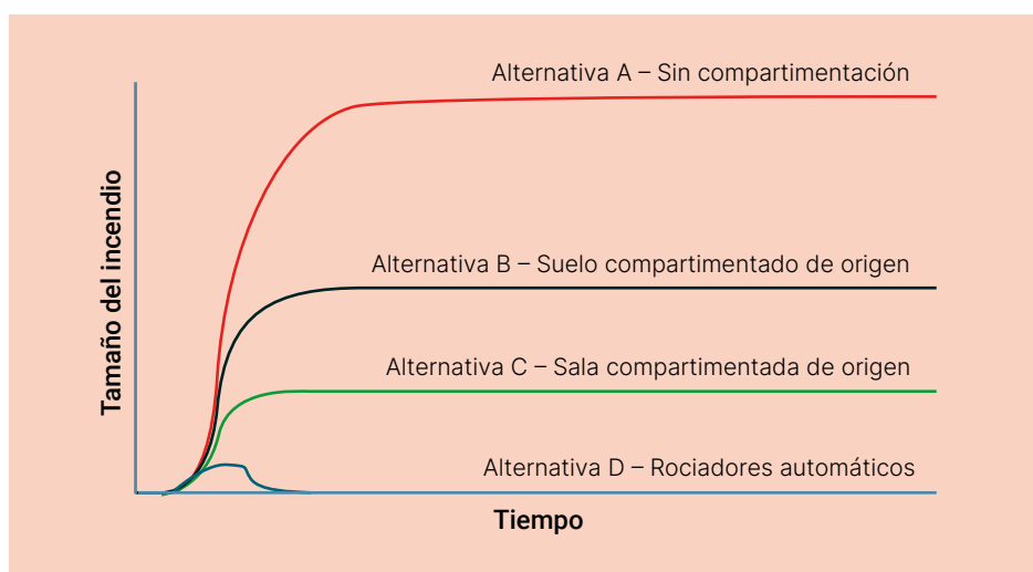
Figura 1. Evaluación de alternativas e impactos en el tamaño del incendio
